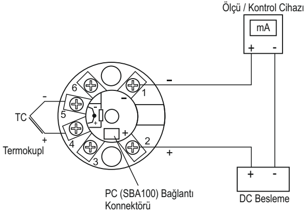
Termokupl Bağlantısı
